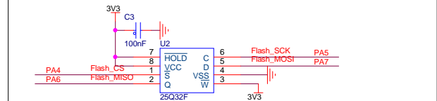
SPI Flash
