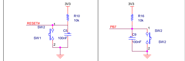
RESET
